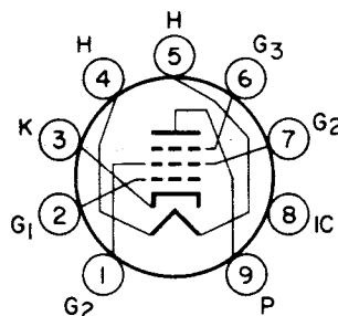
JEDEC 9QU
